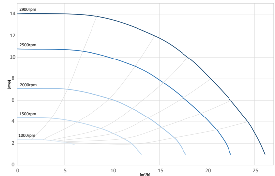
Кривая характеристик EcoVISE
