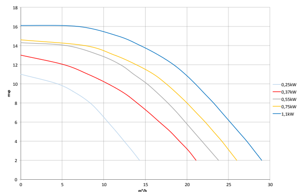
Кривая характеристик WaterVISE / FloVISE
